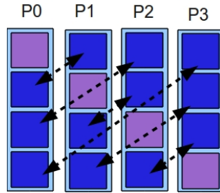
FIGURE A.14 – Représentation bi-dimensionnel de l’algorithme de transposition, impliquant les bâtonnets.
